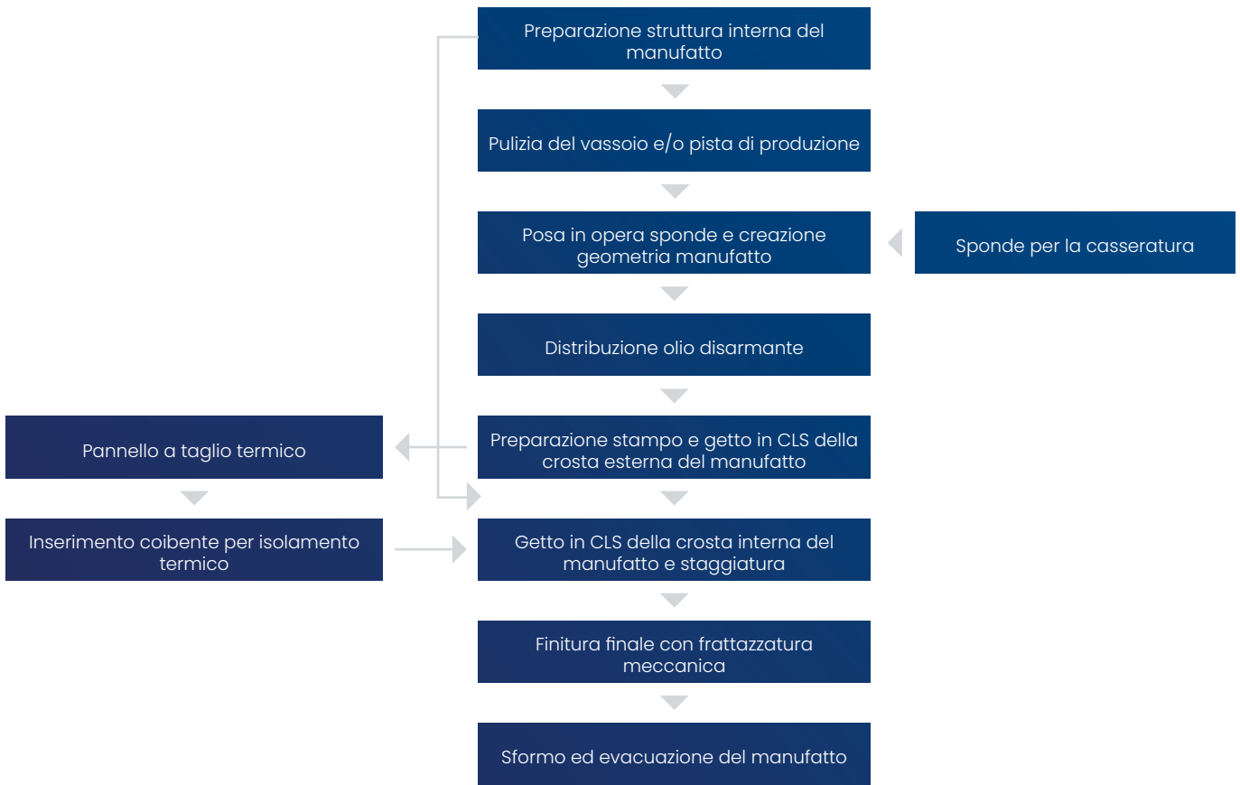
Figura 3: Schema ciclo produttivo pannello prefabbricato Manini
